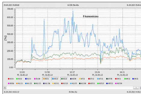
Rys. 4. Dominująca 5. harmoniczna
