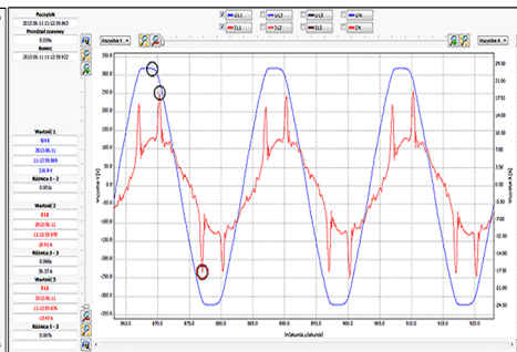
Rys. 8. Przebieg oscyloskopowy prądu i napięcia fazowego podczas działania angiografu
