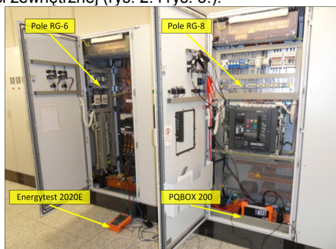
Rys. 1. Widok Rozdzielni Głównej podczas pomiarów
